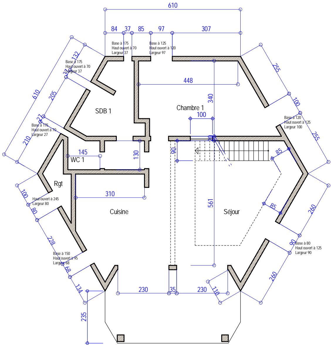
Vue en plan du RDC (coté)
