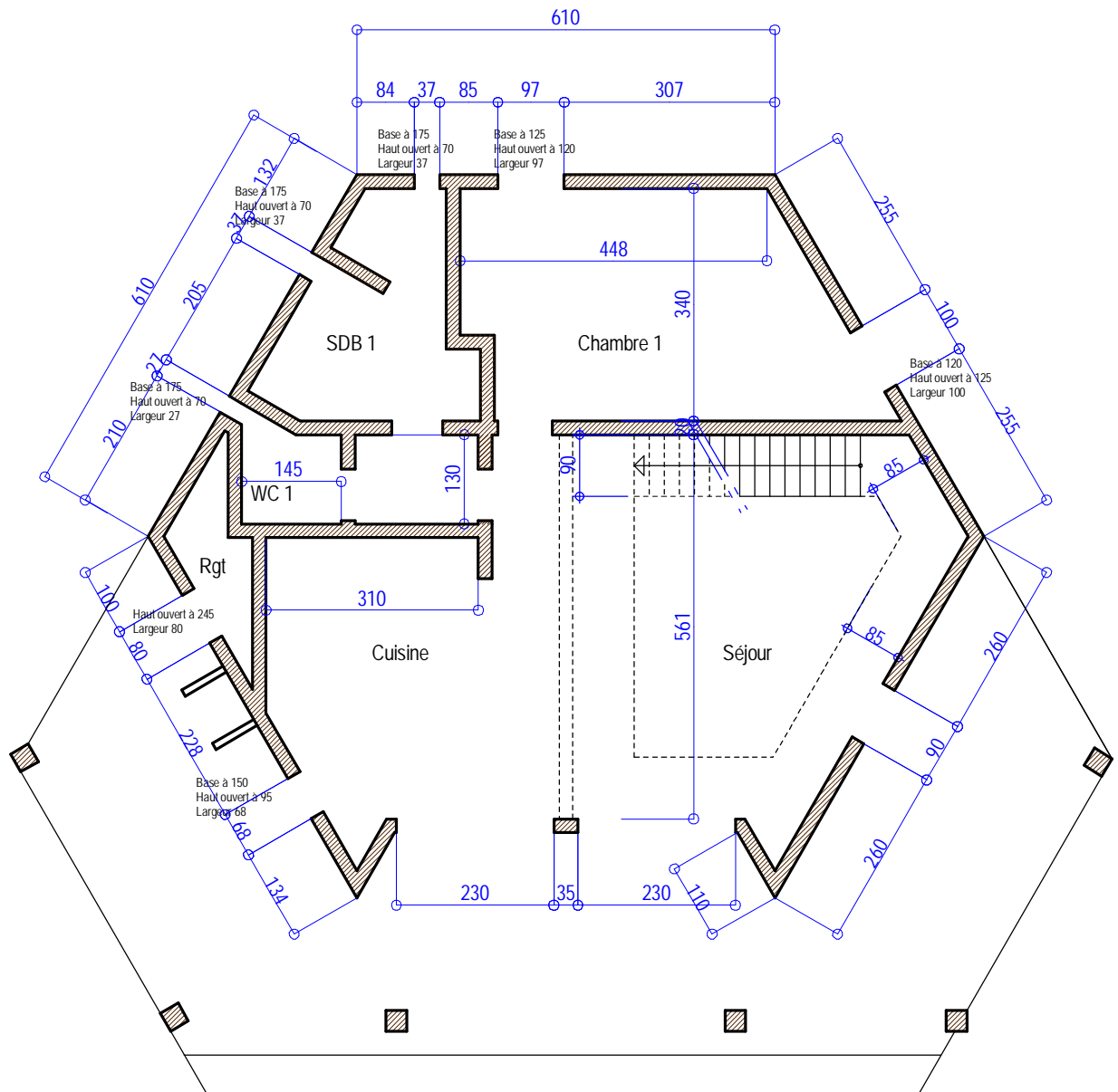
Vue en plan du RDC (coté)
