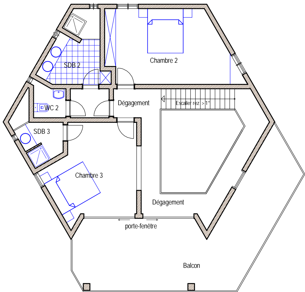
Vue en plan du 1er étage (en mezzanine sur le RDC)
