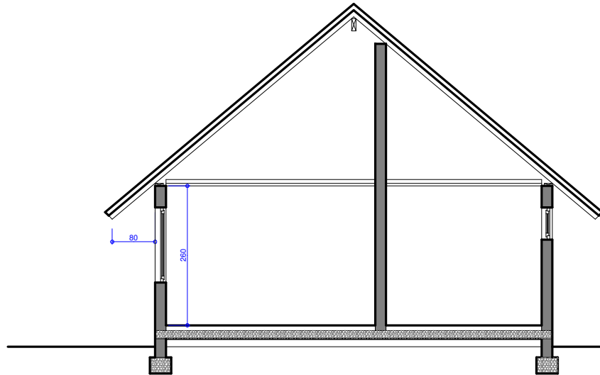
COUPE A-A
